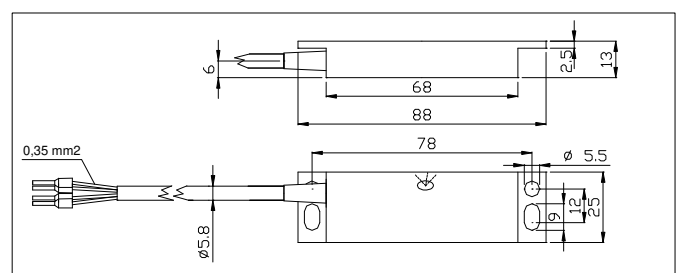
Fig. 4 Dimensions
